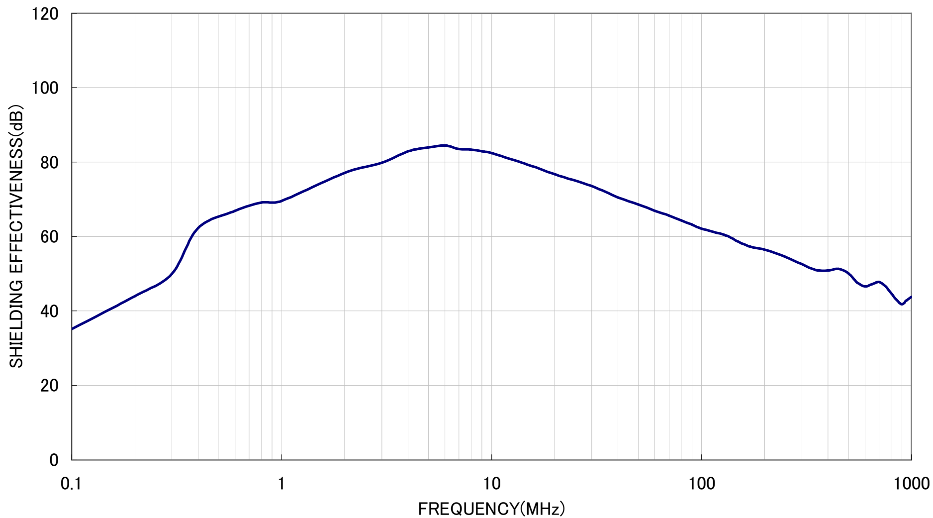
メタックス102C 電界シールドデータ(KEC法)
